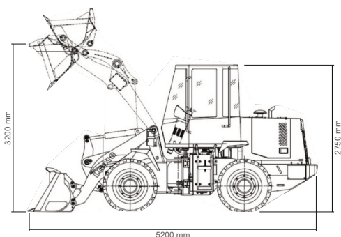
Dimensões principais
