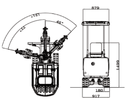
Dimensões em manobras de trabalho
