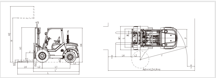
Dimensões principais
