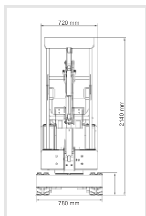
Dimensões principais
